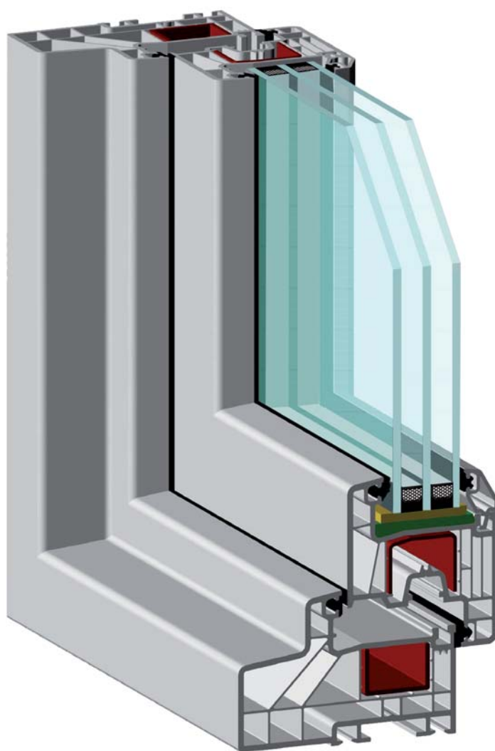
Модификация EXPROF AeroExperta с широкой коробкой серии S571
